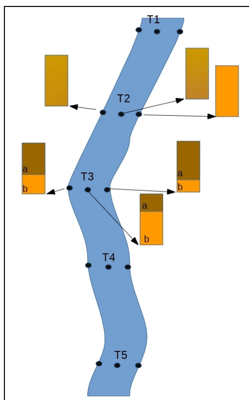
Figura 4 - Piano di campionamento finalizzato alla caratterizzazione dei materiali di scavo in alveo. Nel tratto fluviale interessato dagli scavi sono realizzati dei transeetti posti a distanze di circa 200 m. Ogni transetto è costituito da tre punti di campionamento. A seconda delle caratteristiche stratigrafiche riscontrate da ogni transetto di otterrà un campione composto (caso del T2) oppure in corrispondenza di significative variazioni stratigrafiche più campioni composti relativi ad ogni singolo strato riconosciuto (per il T3 sono considerati due campioni composti relativi rispettivamente allo strato a e allo strato b).
